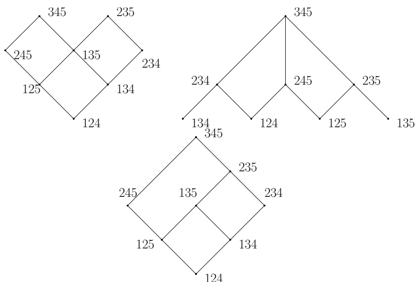
Figure 2: The active orders <_{int} , <_{ext} , and <_{ext/int} , respectively.
